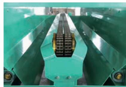
チェーン式前取り装置
